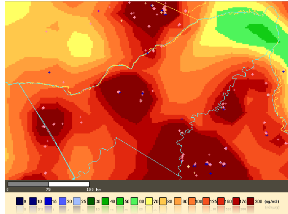
DISTRIBUCIÓN DEL MONÓXIDO DE CARBONO EN LA REGIÓN DE FECHA 18-AGO-2010
